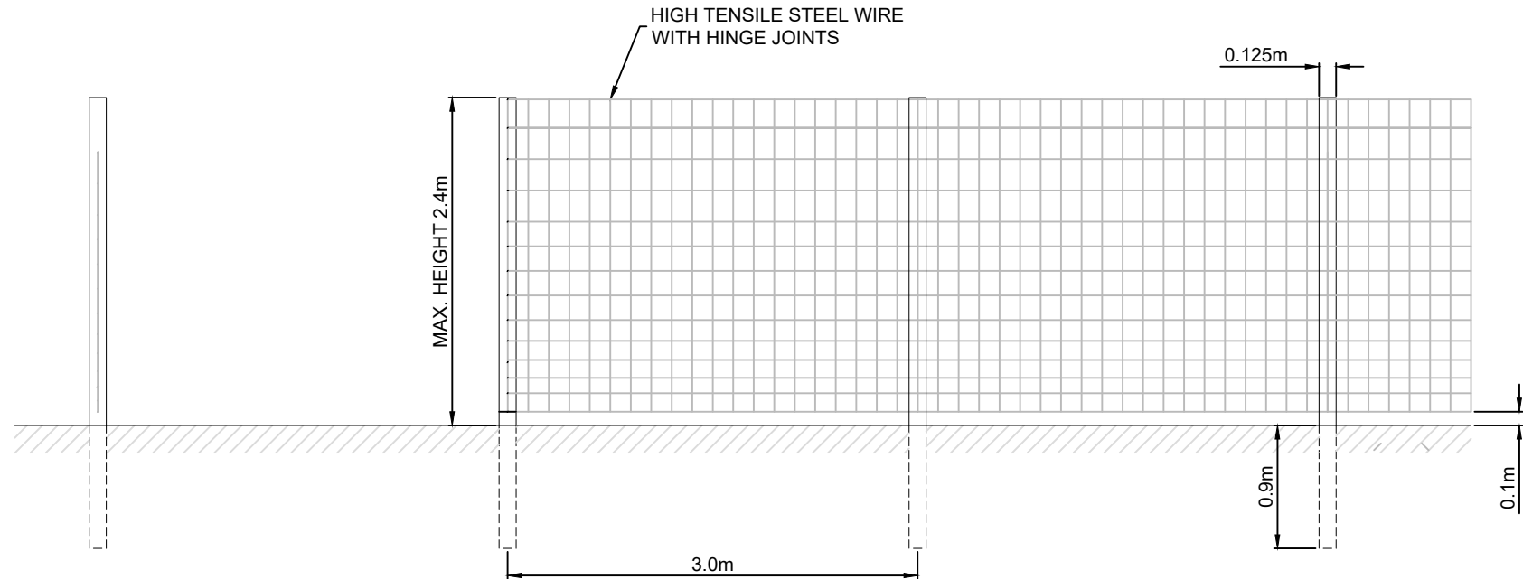
END ELEVATION
